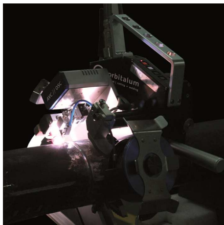
Saldatura orbitale con la serie ORBIWELD TP (Orbitalum) Foto: Orbitalum Tools GmbH
